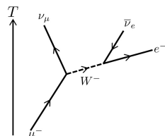
Fig. 3c: Feynman-Diagramm des beobachteten Prozesses (aus Wikipedia)
